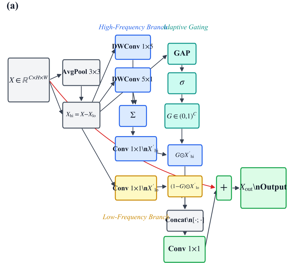
FDDE Module
