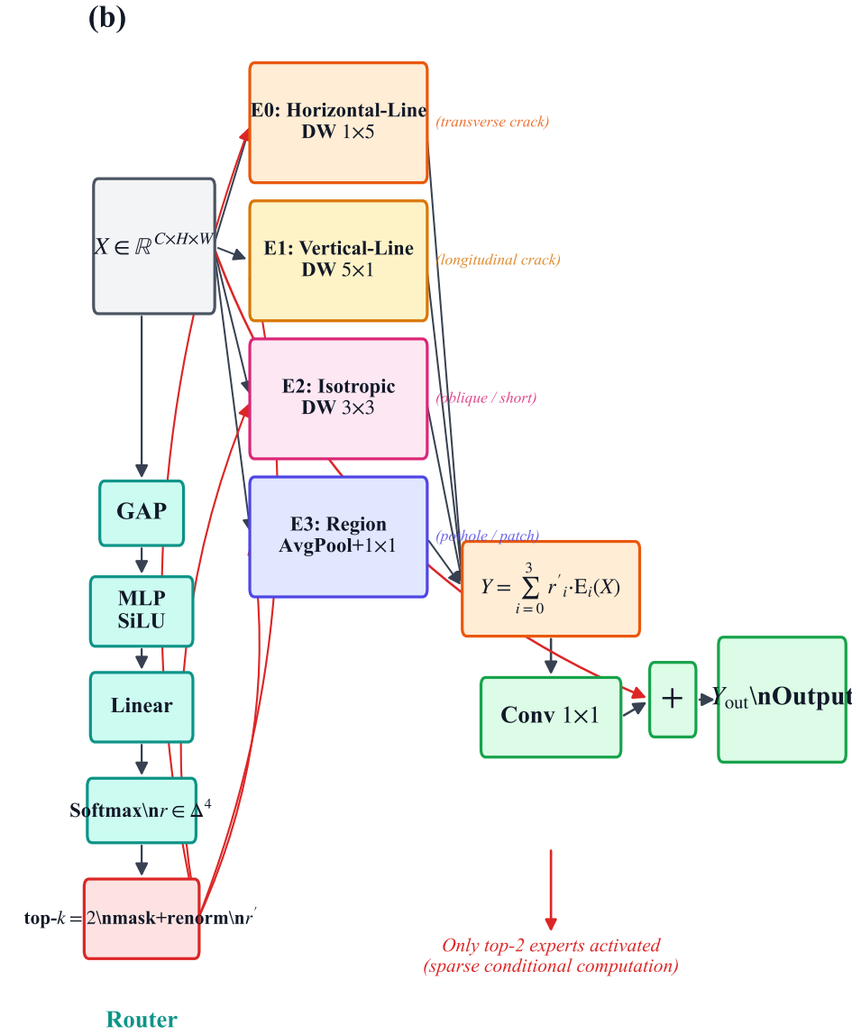
MorphSparseMoE Module
